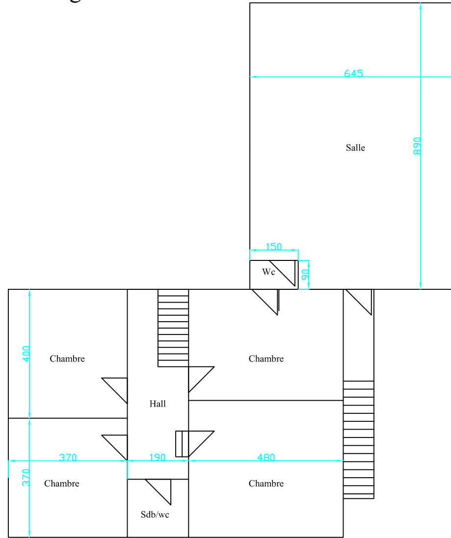
1er étage
